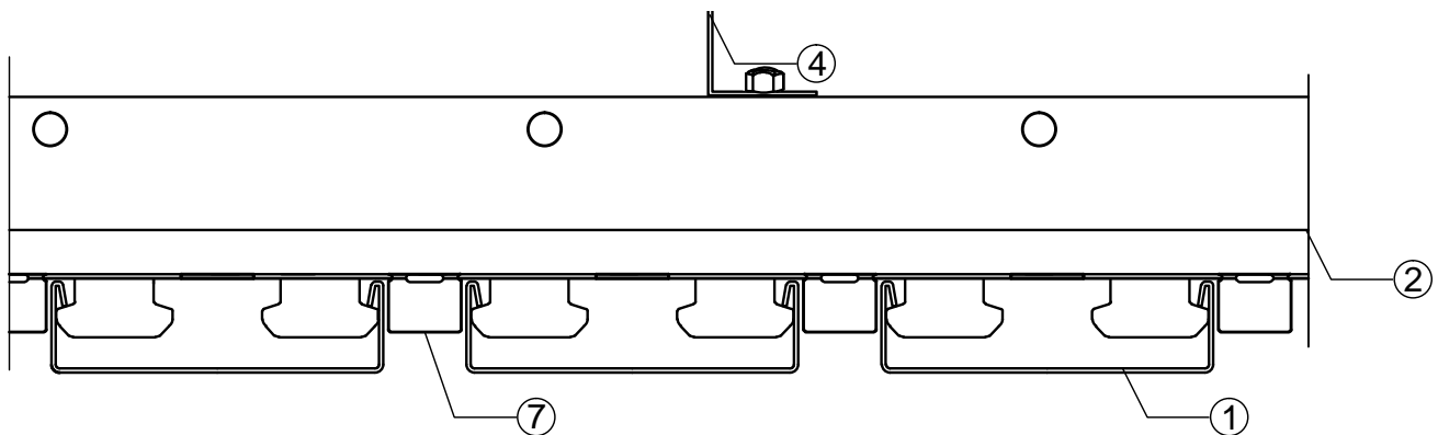
Drucksteife Abhängung mit Noniusunterteilen und Sicherungsstiften
